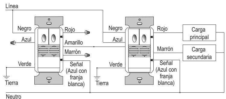
Cableado de dos niveles (DSW-302 – hasta 4 sensores)
